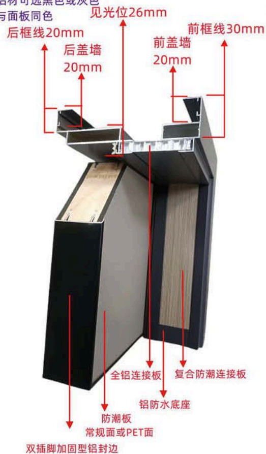
窄边铝木门解剖图
