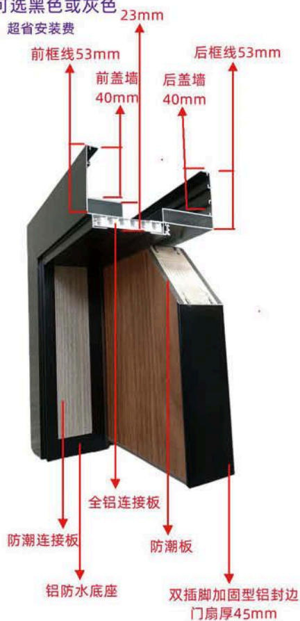
宽边铝木门解剖图
